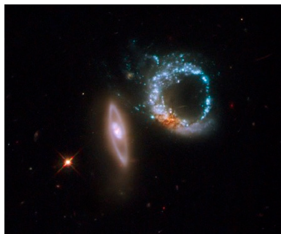
Arp 147
