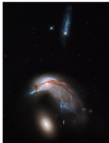
Arp 142
